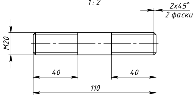
Поз.3 (Шпилька)
