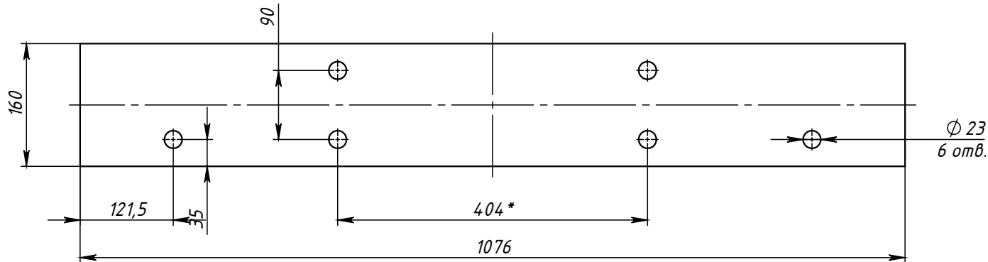
Поз.1 (Полухомут) развертка
